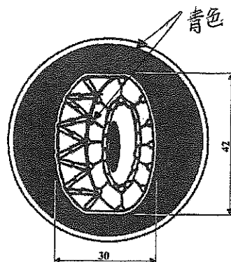
「タイヤチェーンを取り付けていない車両通行止め」(310-3)
